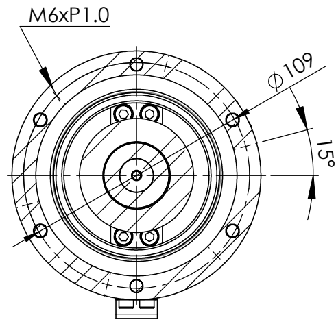
剖面圖 E-E
