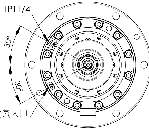
視圖 B
